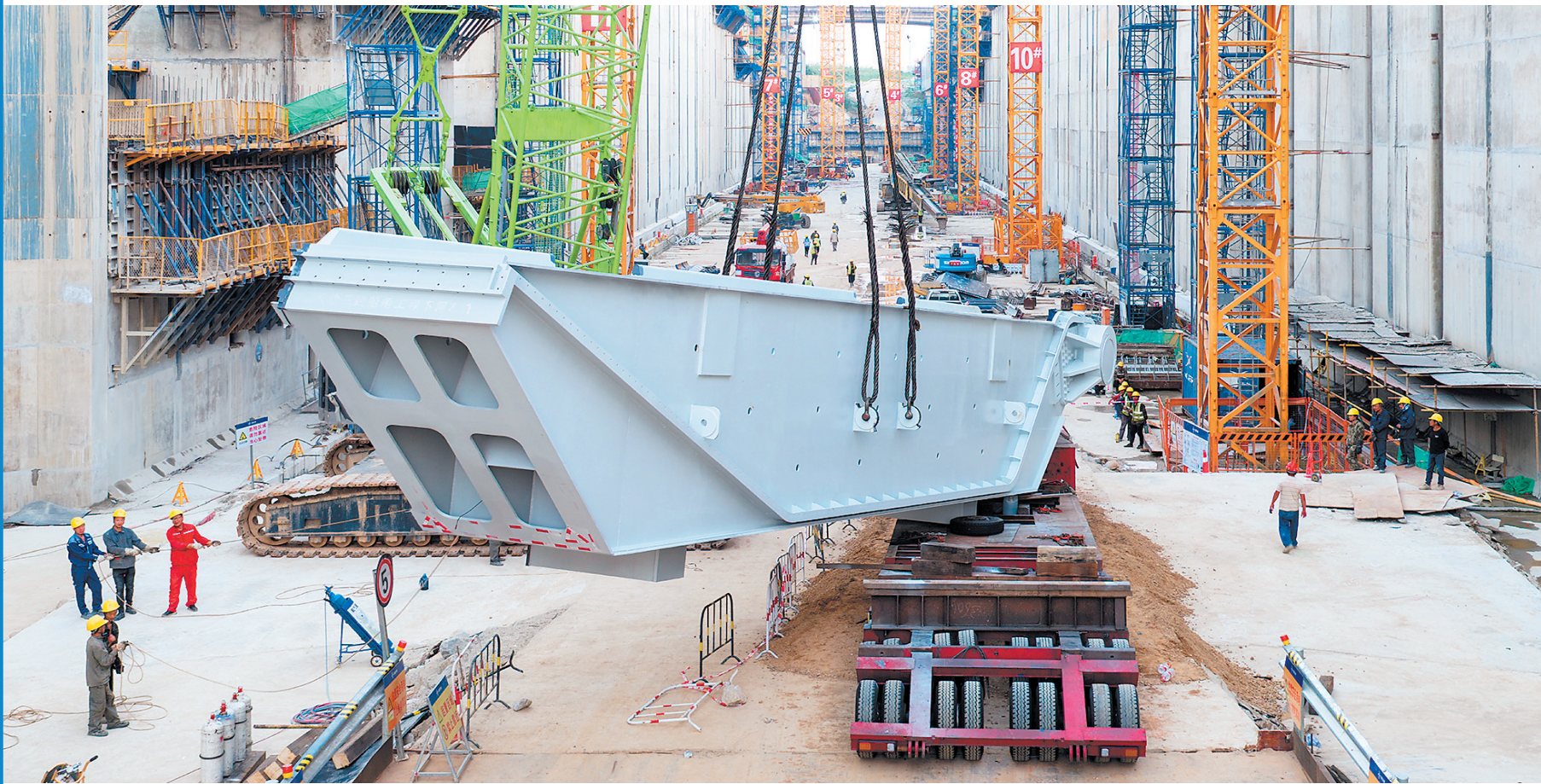
9月10日,由中交四航局承建的湘江长沙综合枢纽三线船闸下闸首人字门首节门叶完成安装。图为吊装过程中。长沙晚报全媒体记者 黄启晴 摄
